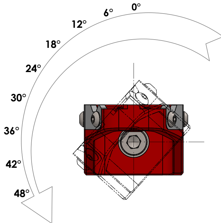
Rotazione pedale - 6 gradi a 8 posizioni Pedal rotation - 6 degrees with 8 positions
