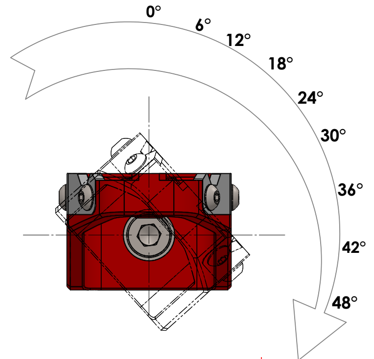
Rotazione pedale + 6 gradi a 8 posizioni Pedal rotation + 6 degrees with 8 positions
